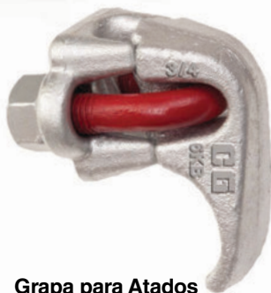
Grapa para Atados "Soft Eye" G-460 (Para usar sin guardacabos)
