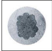
Corte transversal del casquillo prensado
