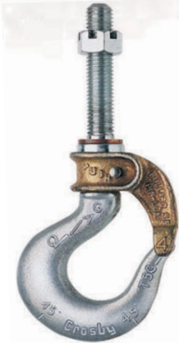
Gancho de Espiga Larga
