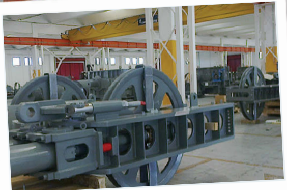
Las poleas forjadas a rodillo producen desempeños notables
